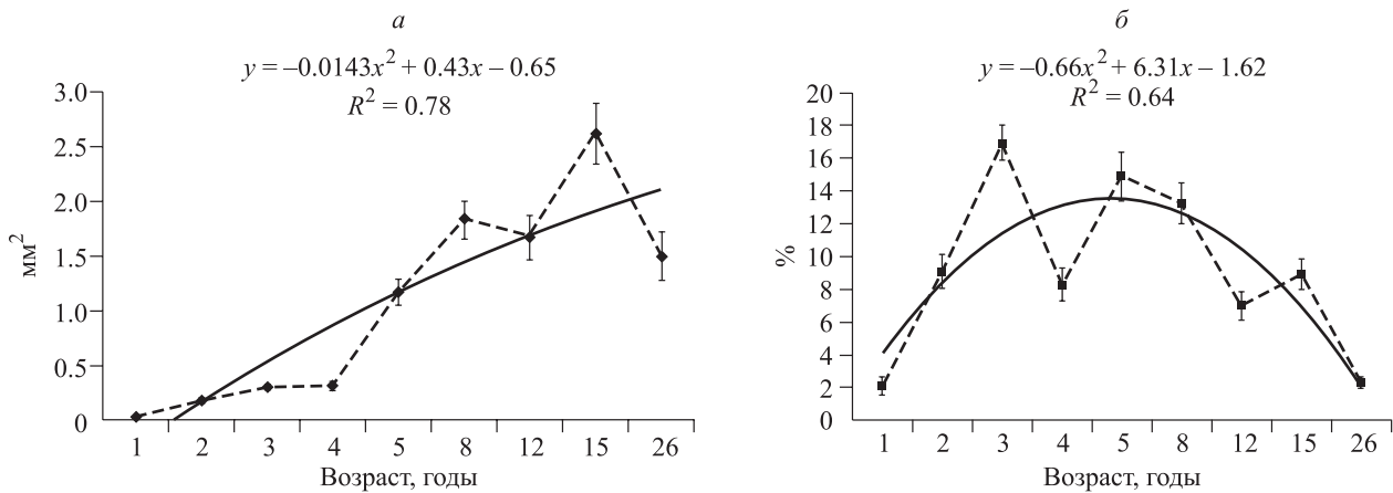
Рис. 3. Развитие тканей аномального строения в онтогенезе стебля спиреи Бовера из кальдеры вулкана Головнина: a – площадь аномальных тканей на поперечном срезе стебля; б – доля площади аномальных тканей на поперечном срезе стебля (от общей площади поперечного сечения стебля).
