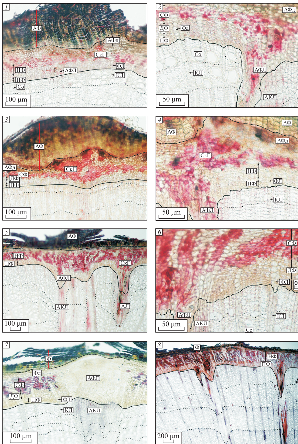
Рис. 2. Структура скелетных стеблей и стволиков спиреи Бовера из кальдеры вулкана Головного (поперечные срезы). 1 – стебель 5–6 лет; 2 – внутренняя часть коры и древесина стебля 5–6 лет; 3 – стебель 7–8 лет; 4 – внутренняя часть коры и древесина стебля 7–8 лет; 5 – стебель 11–12 лет; 6 – внутренняя часть коры и древесина стебля 11–12 лет; 7 – стебель 13–15 лет; 8 – стебель 26–27 лет. ДФ – дилатированная непроводящая флоэма, СФ – склерифицированная непроводящая флоэма. Остальные условные обозначения см. рис. 1. Сплошной черной линией обозначен камбий, пунктирной – феллоген, точечной – границы годичных приростов древесины.
